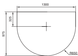
Voor alle modellen zonder zijruit – Draaihoek 90° Plaatstaal Dikte 1,5 mm, grijs of zwart
